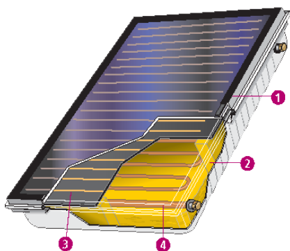
Capteur solaire version verticale
